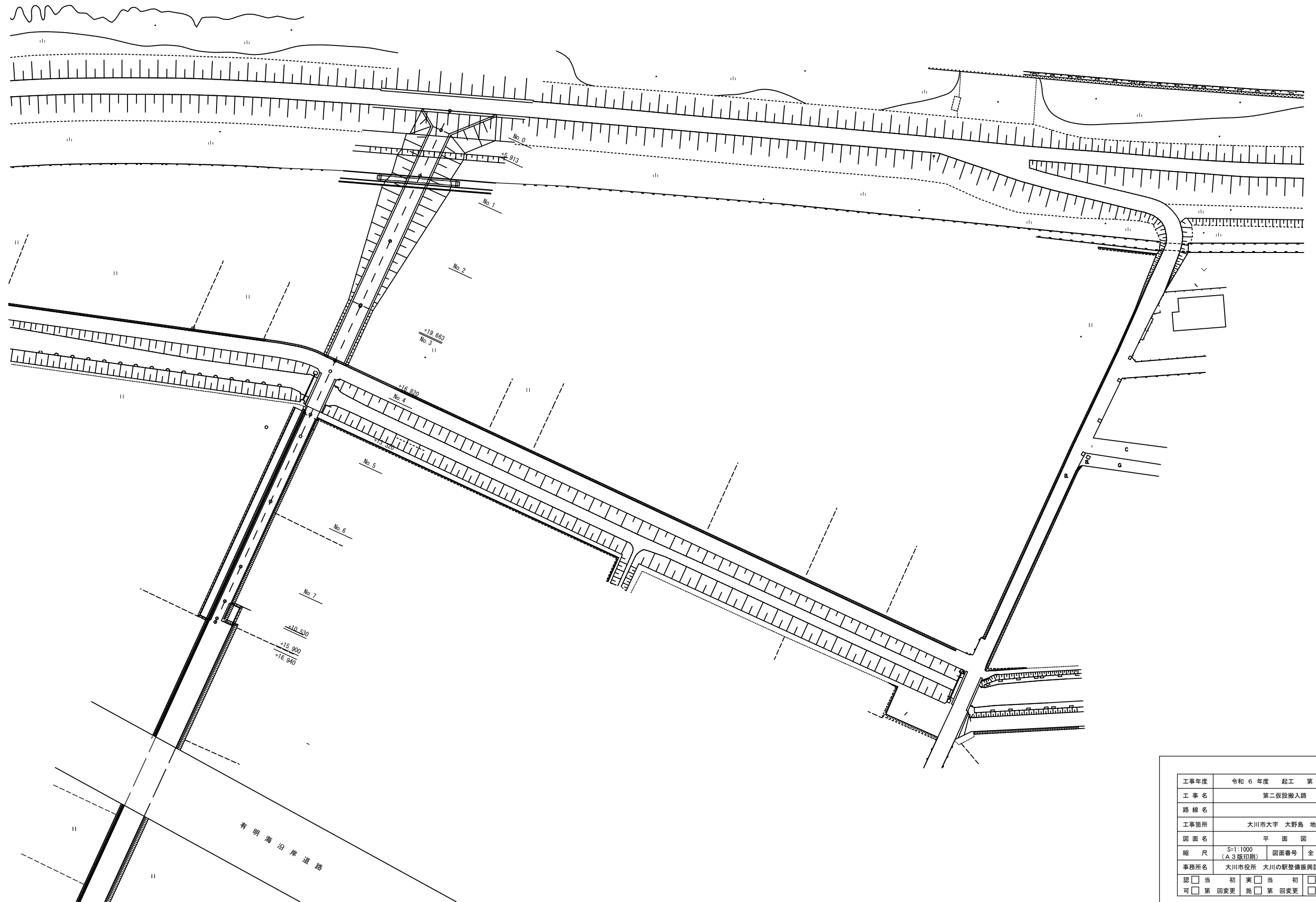
平面図 S=1:1000
